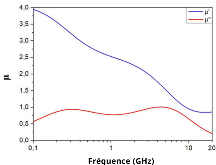
Perméabilité (mesurée)
